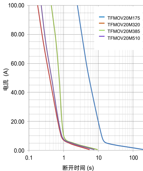
受限电流测试曲线 (UL 1449)
