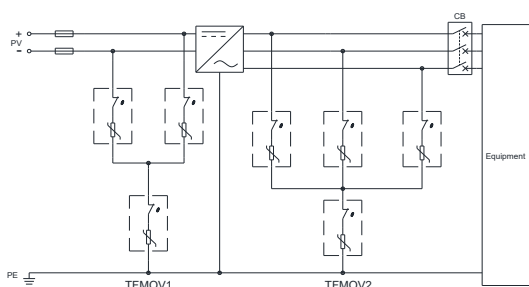
光伏逆变器
