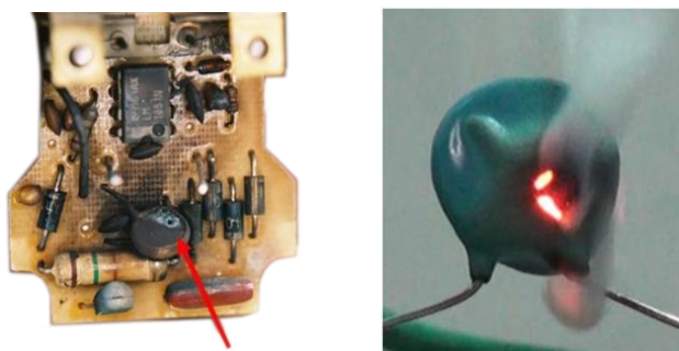
压敏电阻穿孔
