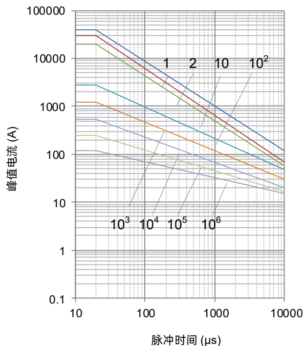
冲击电流降额曲线
